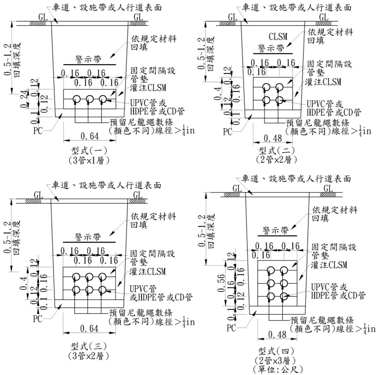
圖 21.3.1 收容性供給管道型式參考圖
